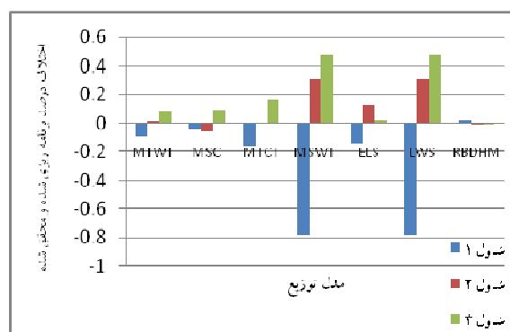
شکل ۳. اختلاف درصد برنامه‌ریزی شده و محقق شده شاول‌ها برای کامیون ۱۰۰ تنی
