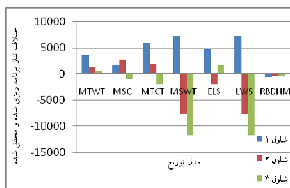
شکل ۴. اختلاف تناژ برنامه‌ریزی شده و محقق شده شاول‌ها برای کامیون ۱۰۰ تنی
