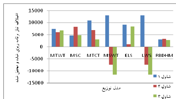
شکل ۱۴. اختلاف تناژ برنامه‌ریزی شده و محقق شده تولید شاول‌ها برای کامیون ۱۵۰ تنی
