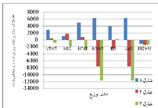
شکل ۷. اختلاف تناژ برنامه‌ریزی شده و محقق شده شاول‌ها برای کامیون ۹۰ تنی
