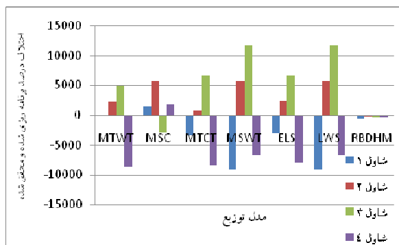
شکل ۱۳. اختلاف درصد برنامه‌ریزی شده و محقق شده تولید شاول ۴
