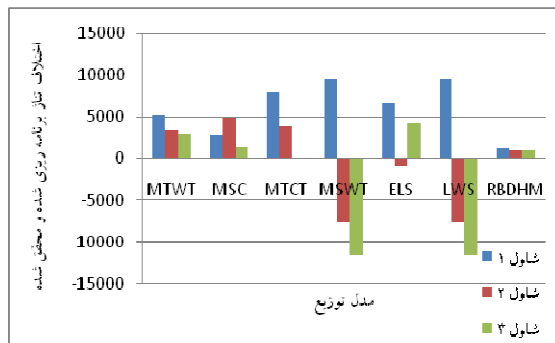
شکل ۱۱. اختلاف درصد برنامه‌ریزی شده و محقق شده تولید شاول‌ها برای کامیون ۱۲۰ تنی
