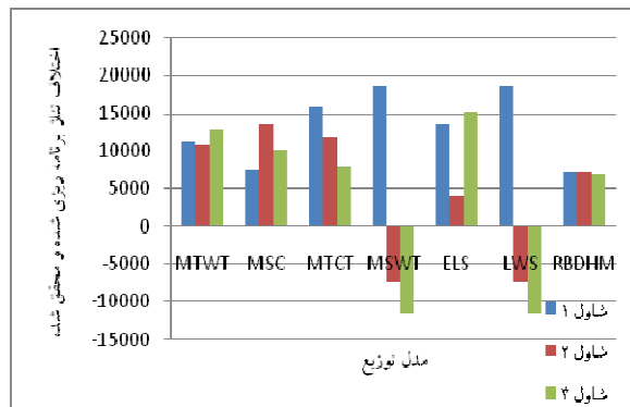
شکل ۱۰. اختلاف تناژ برنامه‌ریزی شده و محقق شده تولید شاول‌ها برای کامیون ۲۰۰ تنی
