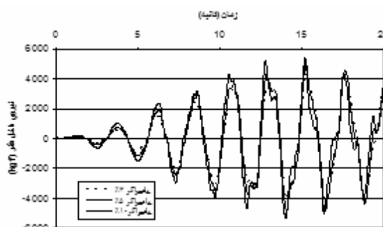
شکل ۱۶. مقدار نیروی فنر در سازه نامیرا تحت زلزله منجیل
