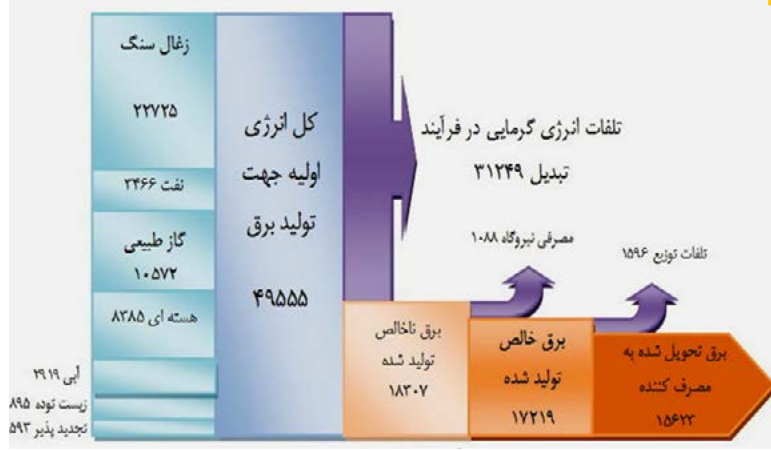
شکل ۱- نمودار جریان انرژی جهانی جهت تولید برق (میلیون تن معادل تفت خام)
